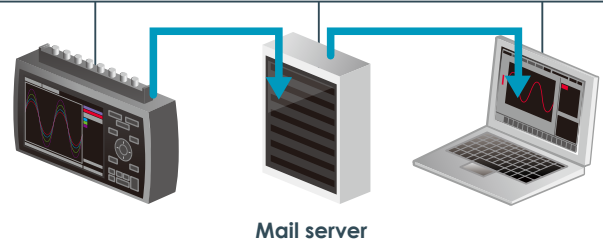
LAN (Ethernet)
